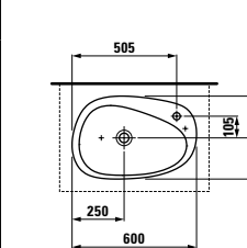
1680.3 Bowl with tapbank Aufsatz-Waschtisch mit Armaturenbank Lavabo avec plage pour la robinetterie Bacinella con banco rubinetteria
