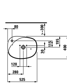
1180.3 Freestanding washbasin Freistehender Waschtisch Lavabo indépendant Lavabo centro stanza
