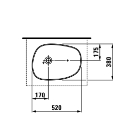
1680.2 Bowl Aufsatz-Waschtisch Lavabo à poser Bacinella
