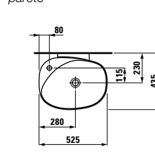
1180.4 Freestanding washbasin with wall-connection Freistehender Waschtisch mit Wand-anbindung Lavabo, indépendant, avec raccordement au mur Lavabo centro stanza con connessioni a parete
