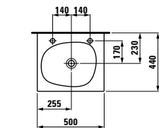
1780.1 Countertop washbasin Waschtisch, unterbaufähig Lavabo à poser sur meuble Lavabo consolle
