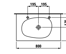
1780.4 Countertop washbasin Waschtisch, unterbaufähig Lavabo à poser sur meuble Lavabo consolle
