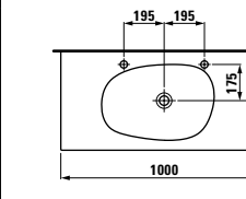
1780.6 Countertop washbasin Waschtisch, unterbaufähig Lavabo à poser sur meuble Lavabo consolle
