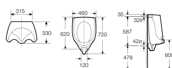
Mural 莫纳 353451..0 后进水
