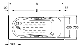
Malibu 马里布 231650..1 带扶手 (1700x750mm) A B L/升 231070..1 带扶手 (1600x750mm) 1700 1513 185 247375..1 带扶手 (1500x750mm) 1600 1413 171 247375..1 带扶手 (1500x750mm) 1500 1313 165
