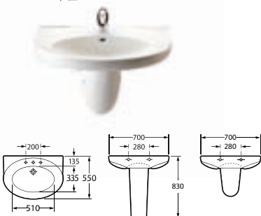
洗脸盆 327412..0 洗脸盆(700x550) 337410..0 立柱 337412..0 半柱
