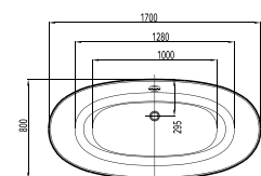
Virginia 维吉亚 248215..0 (1700x800mm)
