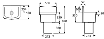
Hamito 汉密顿 371457..0 拖布池 371458..0 立柱
