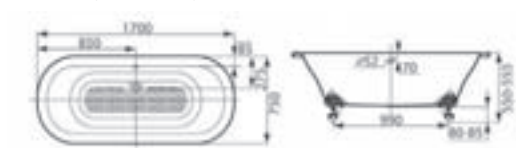
Faro 菲洛独立式 2N076B..0 (1700x750mm) / 291094000 镀铬鹰脚
