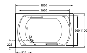
Thalassa 德拉 247580..1 /247579..1 (1850x1100mm)
