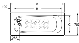
Continental 康婷 212911..1 (1700x700mm)/212912..1 (1600x700mm) A B C L/升 212913..1 (1500x700mm)/212914..1 (1400x700mm) 1700 1530 570 182 211516..1 (1200x700mm) 1600 1430 570 170 1500 1330 570 161 1400 1230 560 144 1200 1050 550 117
