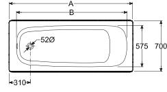
Contesa 康莎 2358A0..0 (1700x700mm) A B L/升 2359A0..0 (1600x700mm) 1700 1525 195 2360A0..0 (1500x700mm) 1600 1425 180 1500 1325 165
