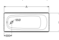
Contesa Plus 康莎 (3.5mm厚) 237760..0 (1700x700mm) A B L/升 237360..0 (1600x700mm) 1700 700 195 1600 700 180
