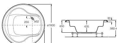
Waikiki 威凯独立式 (1600x1600mm) 248232..0 / 248233..0 带扶手 (1600x1600mm)
