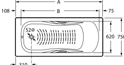
Princess-n 普林 220270..1 带扶手 (1700x750mm) A B L/升 220370..1 带扶手 (1600x750mm) 1700 1517 215 220470..1 带扶手 (1500x750mm) 1600 1417 205 1500 1317 190
