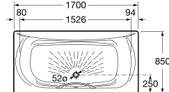
Akira 阿其拉 232570..R 带扶手 (1700x850mm)
