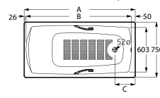
Mykonos 麦克罗 2N0160..0 不带扶手 (1700x750mm) A B C L/升 2N0170..1 带扶手 (1700x750mm) 1500 1424 275 162 2N0360..0 不带扶手 (1500x750mm) 1700 1624 285 190 2N0370..1 带扶手 (1500x750mm)
