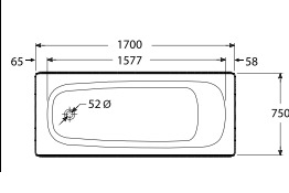
Body Plus 博迪 (3.5mm厚) 237950..0 (1700x750mm)
