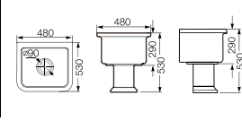
Hamito-S 汉密顿-S 37145500 拖布池 37145600 立柱
