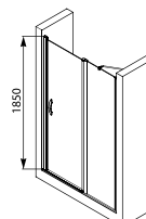
Non-standard 转轴式非标淋浴房 N107L0012 左开门 1固1活 N107R0012 右开门 1固1活 适做范围: (1000-1500) x 1850
