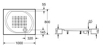
DAIQUIRI 黛奇方型 276015..0 (1000x800mm)
