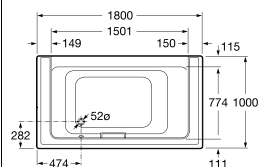
America 艾美 247552..1 带扶手 (1800x1000mm)
