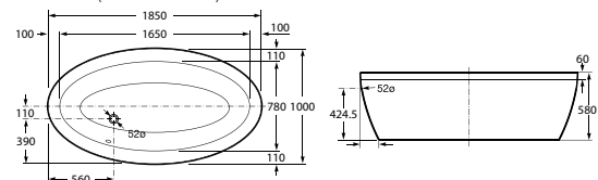
Georgia 乔治亚独立式 247977..1 (1850x1000mm)
