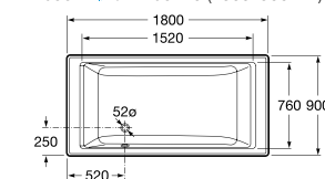
Vythos 韦德 247593..1 /247592..0 (1800x900mm)
