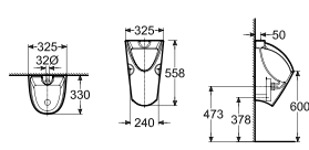
Chic 启克 359451..0 上进水
