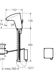
M2 摩图单冷 5A5655C0N 电池供电 5A5755C0N 交流电
