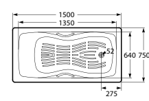
Corfu 科芙 2N0660..0 不带扶手 (1500x750mm) 2N0670..1 带扶手 (1500x750mm)
