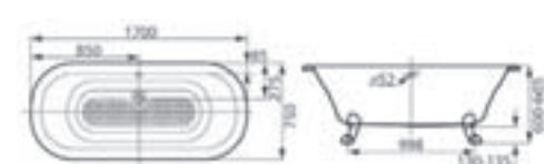
Faro 菲洛独立式 2N1060..0 (1700x750mm) / 291069001 镀铬老虎脚
