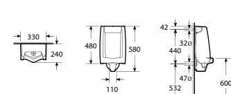
Bana-S 班纳-S 359454..0 后进水
