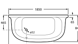
Frontalis 梵钛立 247717..1 (1850x 840mm)
