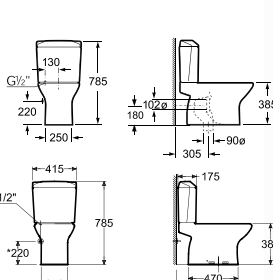
座厕(地排坑距400mm或横排) 3424B1..0 底座 3414A0..0 水箱连水箱配件 80N410..1 欧乐盖板(标准配置) 80N412..1 欧乐阻尼盖板
