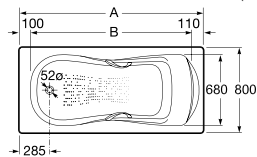
Haiti 海蒂 247279..1 带扶手 (1700x800mm) A B L/升 247284..1 带扶手 (1600x800mm) 1700 1490 190 247601..1 带扶手 (1500x800mm) 1600 1390 180 247601..1 带扶手 (1500x800mm) 1500 1290 168
