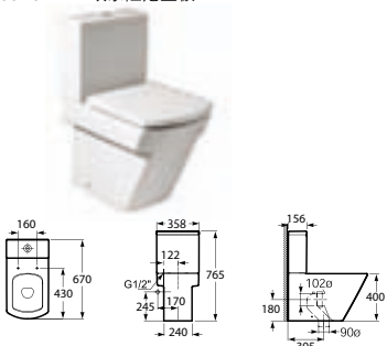
座厕(地/横排水双用, 地排坑距305mm) 3424B7..0 底座 / 3414B6..0 水箱连水箱配件 80N626..1 欧乐盖板(标准配置) 80N622..1 欧乐阻尼盖板
