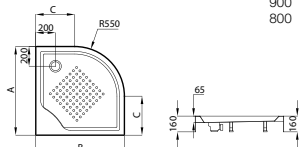
SHERRY 秀丽角型 带扶手 276020..0 / 276016..0 / 276021..0
