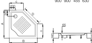
BRANDY 白兰地钻石型 276017..0 / 276022..0
