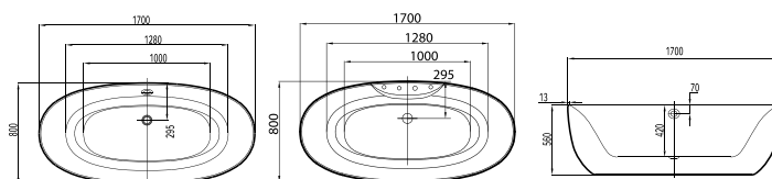
Virginia 维吉亚独立式 248217..0 (1700x800mm) / 248218..0 (带缸边龙头) (1700x800mm)
