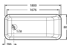
Element 伊元素 247704..0 (1800x800mm)
