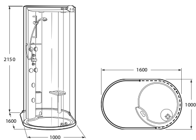
2H0240000 按摩淋浴房
