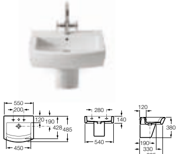
洗脸盆 327881..0 (550x485) 32788H..0 三孔(550x485) 337621..0 半柱
