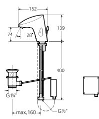
M2 摩图冷热水 5A5355C0N 电池供电 5A5555C0N 交流电
