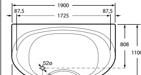
Veranda 华兰 247357..1 带扶手 (1900x1100mm)
