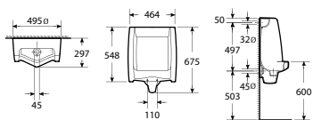
Bana 班纳 359455..0 后进水
