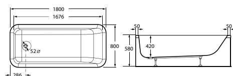
Element 伊元素独立式 247976..1 (1800x800mm)
