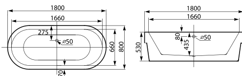
Ibiza 艾比莎独立式 26N007..0 (1800x800mm)
