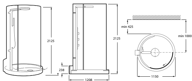
2H0392120 自动开门淋浴房
