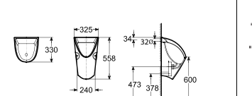
Chic 启克 35945J..0 后进水
